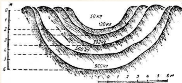
Рис. 22. Действие американских фугасных бомб:
